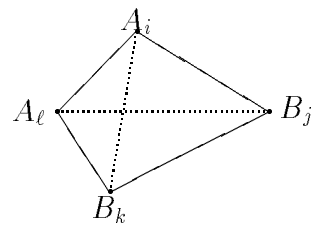
Figure 2: l'inégalité du quadrangle convexe
