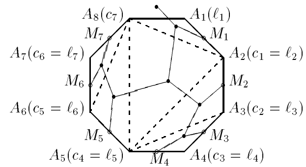
Figure 1: octogone et produit matriciel
